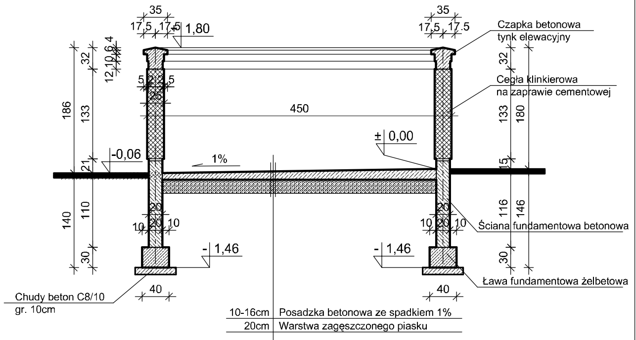
PRZEKRÓJ 1-1
