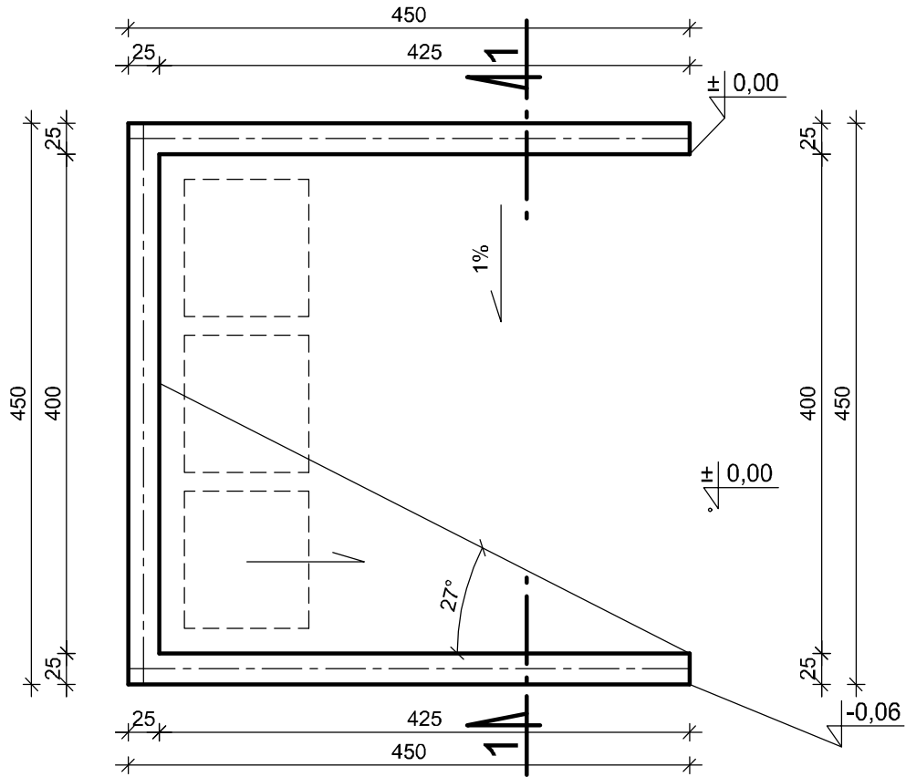
PRZEKRÓJ POZIOMY
