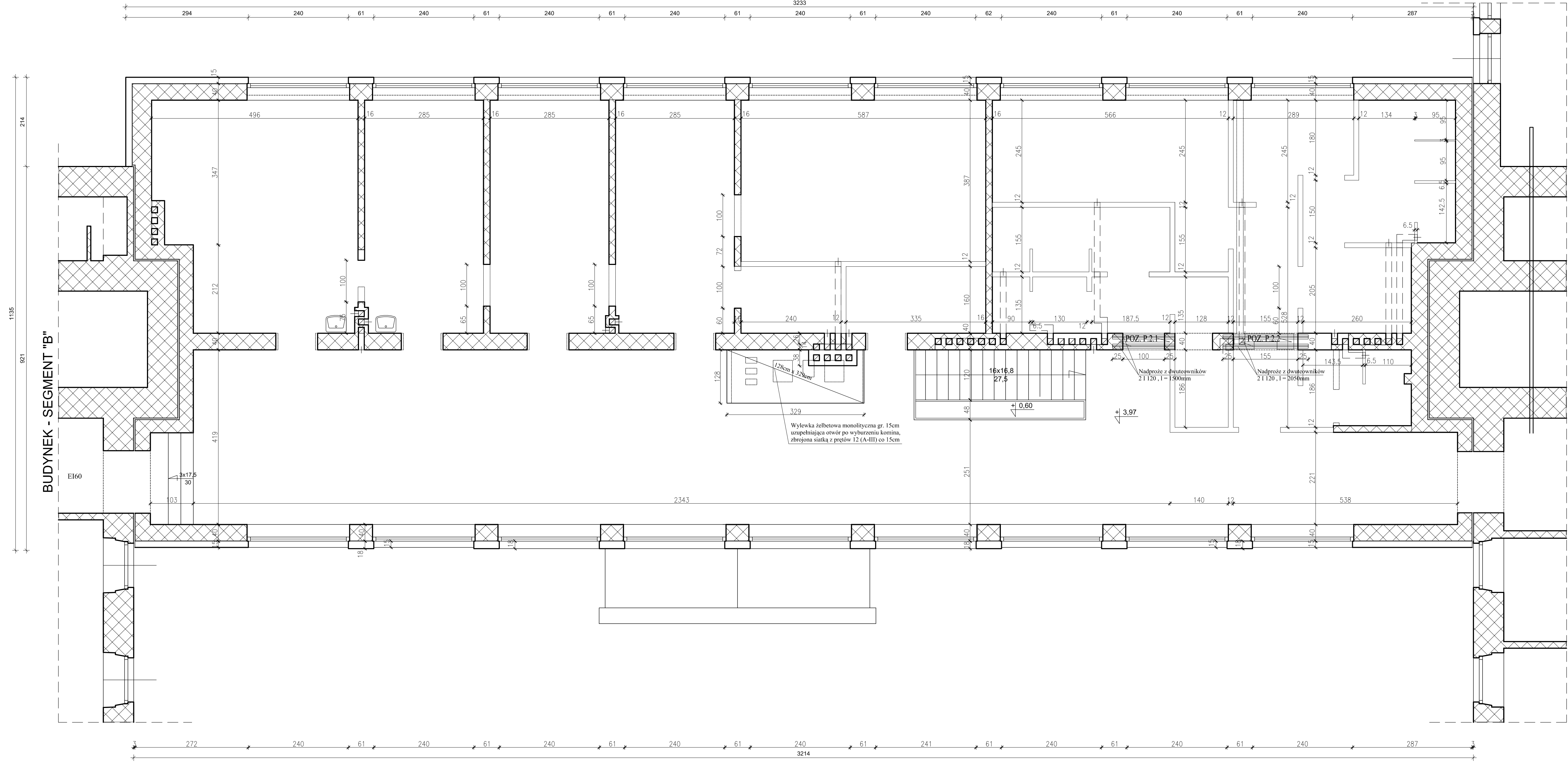
UKŁAD KONSTRUKCYJNY PIĘTRA Segment "A" Skala 1:50
