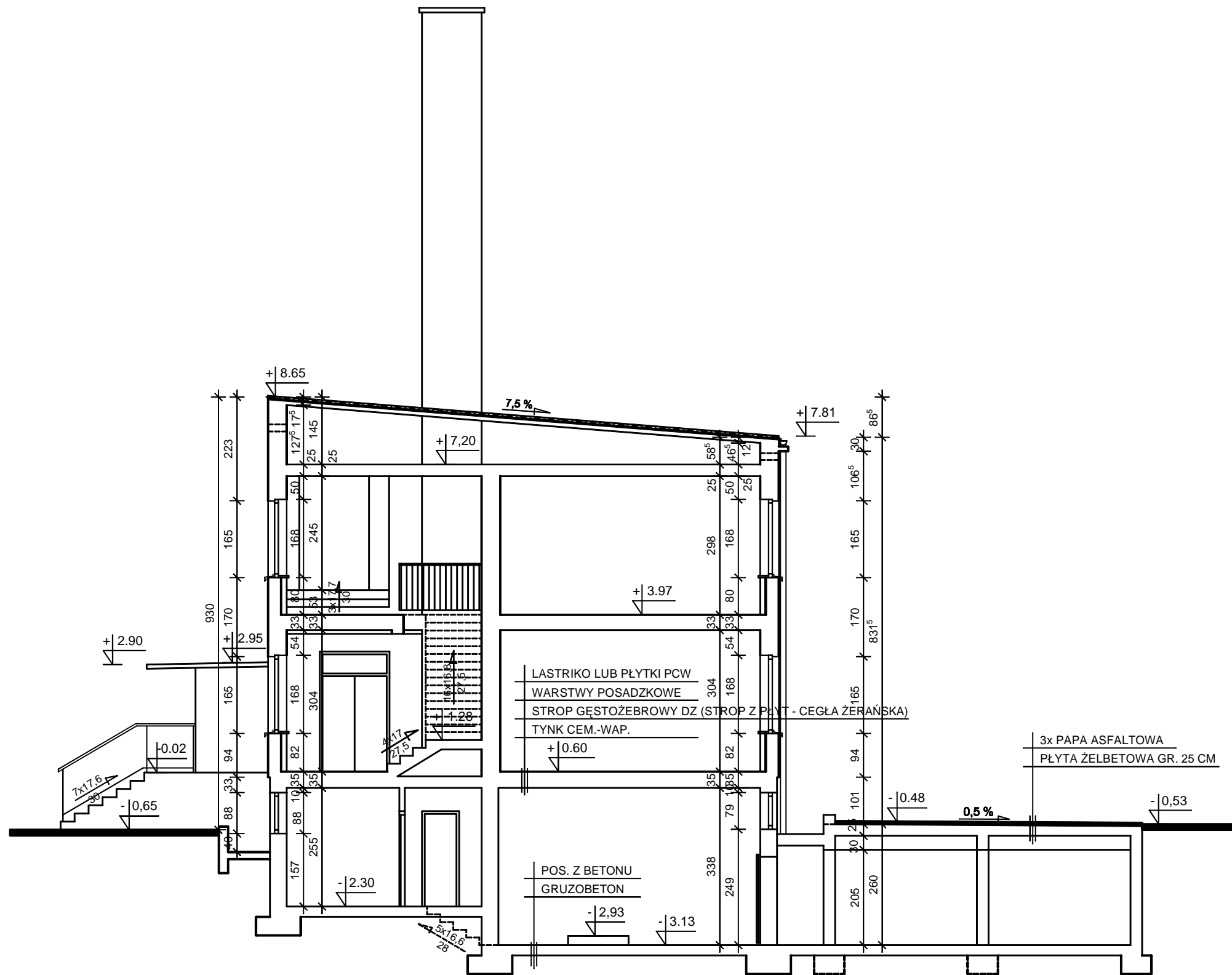
PRZEKRÓJ PIONOWY 3-3
